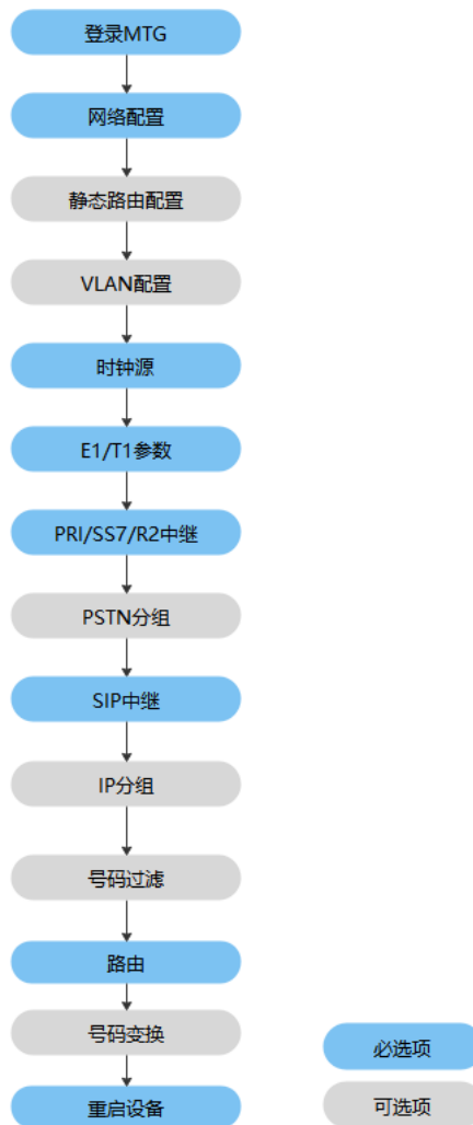
图2-2-4配置流程
