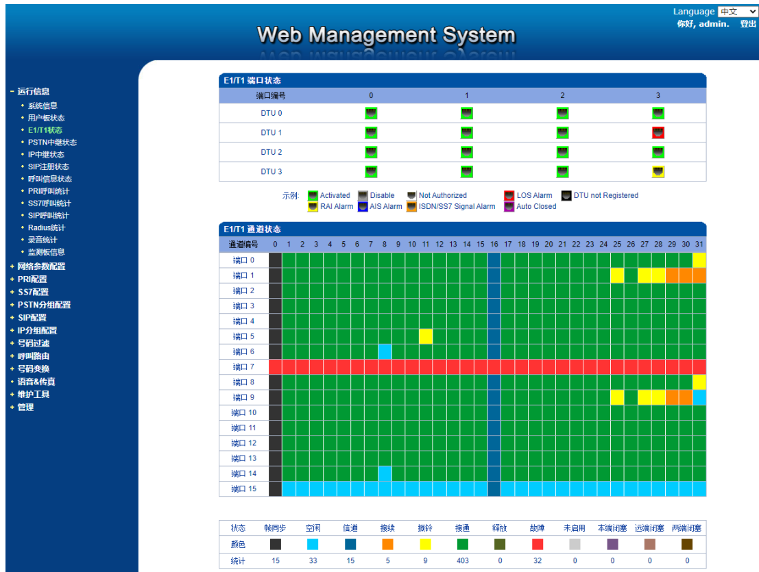
图2-3-5 E1/T1状态
